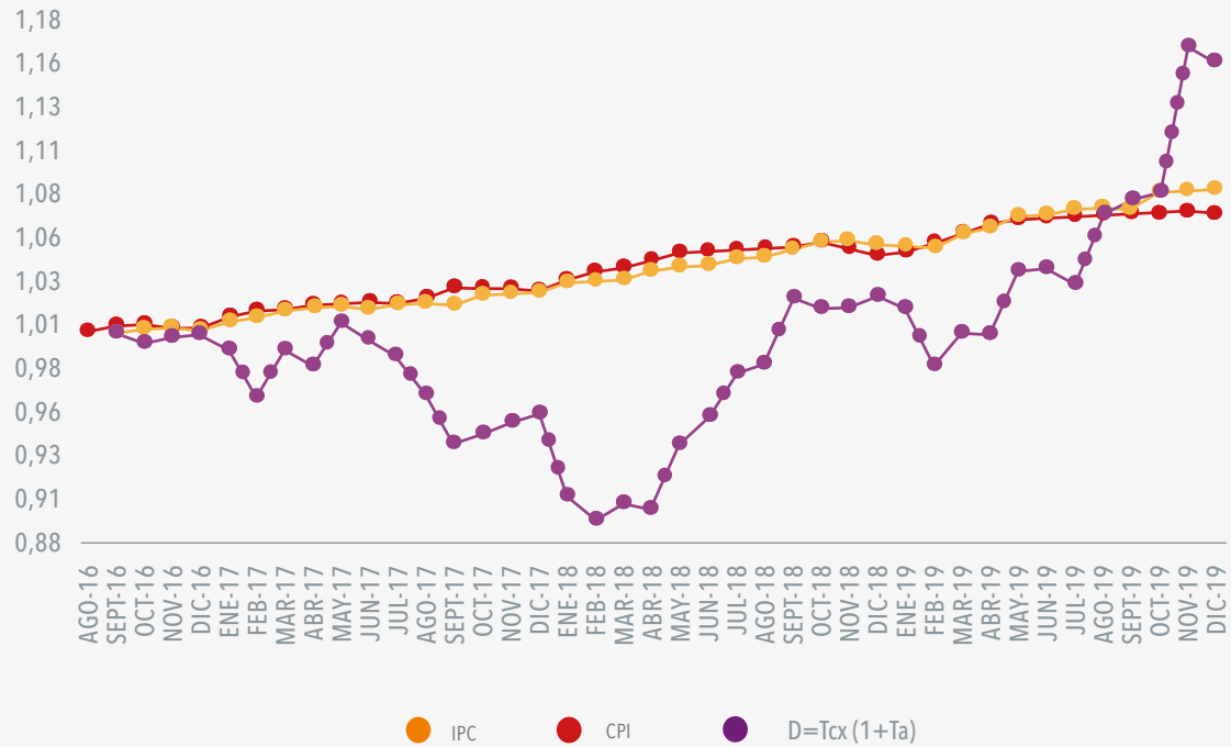
GRÁFICO 28 EVOLUCIÓN PARÁMETROS DEL VAD
