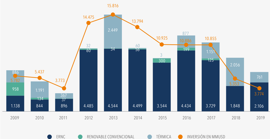
GRÁFICO 8 EVOLUCIÓN DE PROYECTOS DE GENERACIÓN ELÉCTRICA CON RCA APROBADA EN MW Y MMUSD
