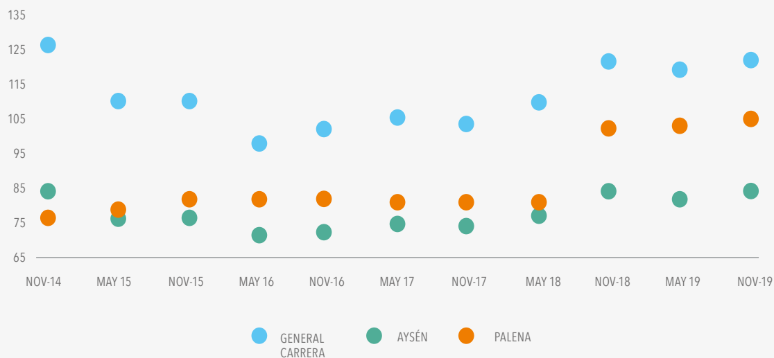
GRÁFICO 25 EVOLUCIÓN DEL PRECIO MONÓMICO DE AYSÉN -PALENA- GENERAL CARRERA EN $/kWh
